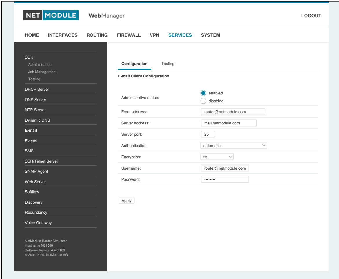
Abbildung 5.42.: E-Mail-Einstellungen
