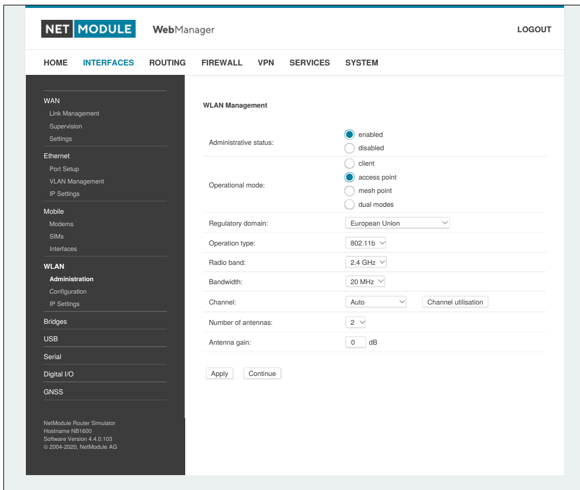
Abbildung 5.14.: WLAN-Verwaltung
