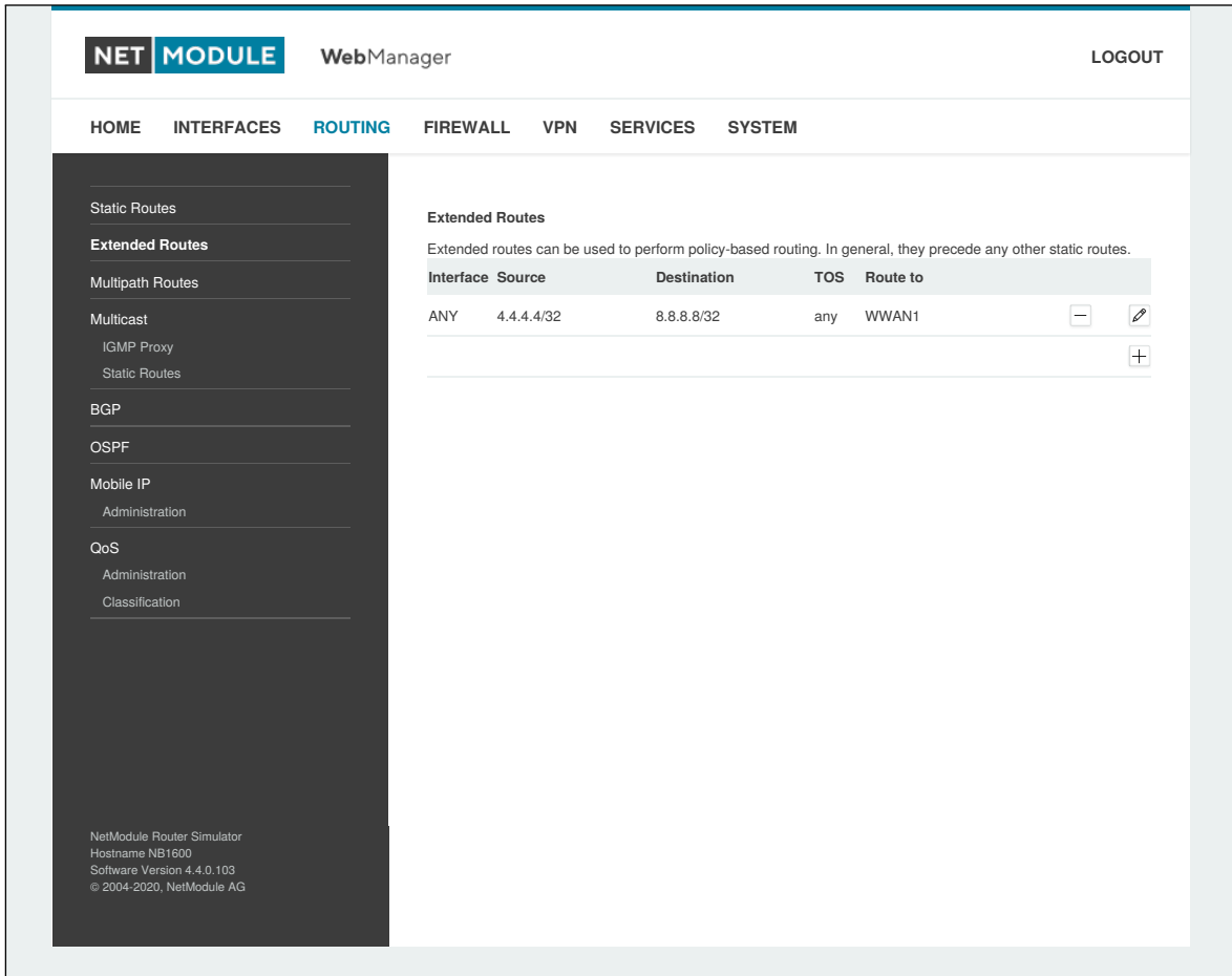
Abbildung 5.23.: Erweitertes Routing
