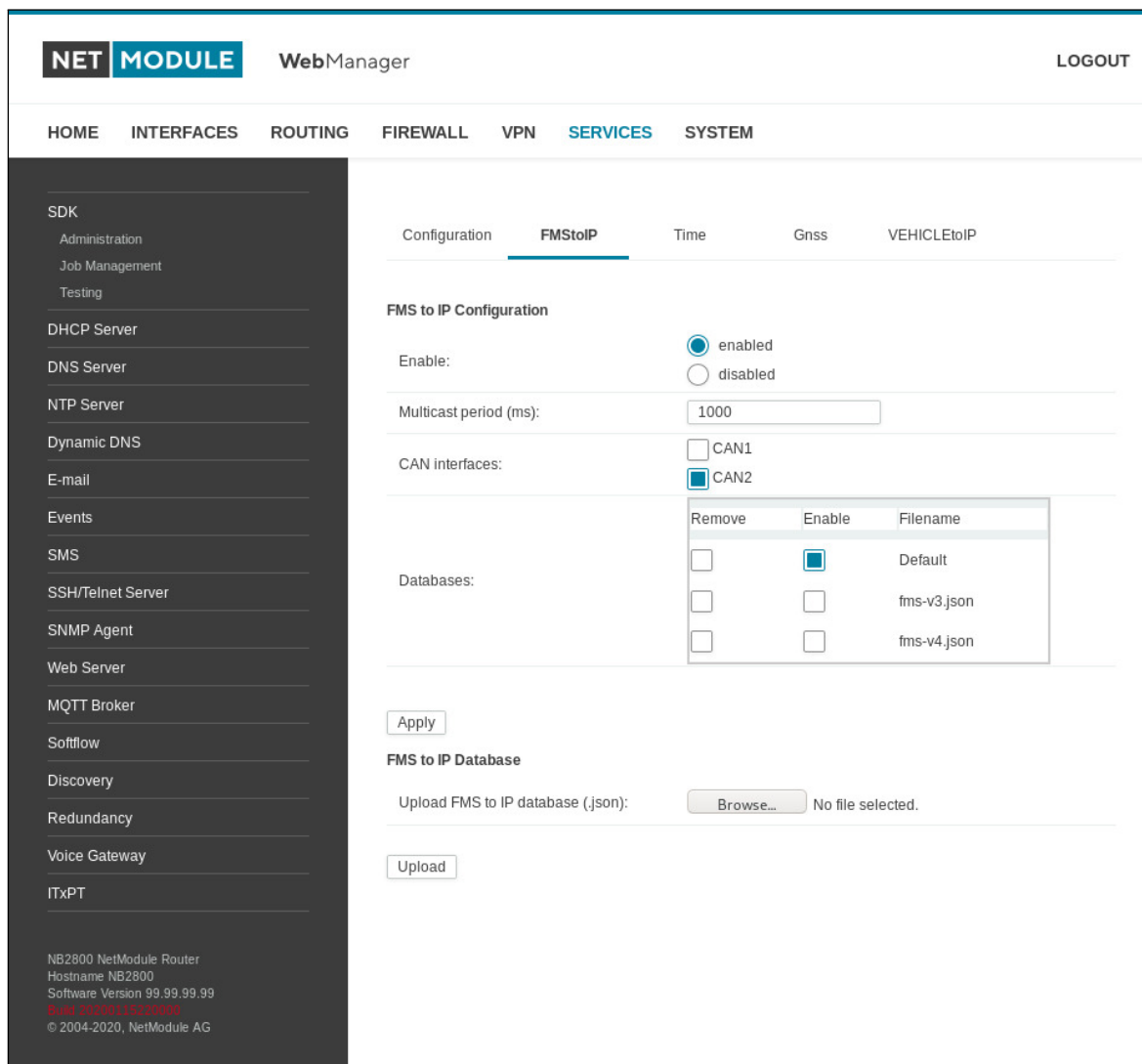
Abbildung 5.49.: ITxPT FMS-to-IP
