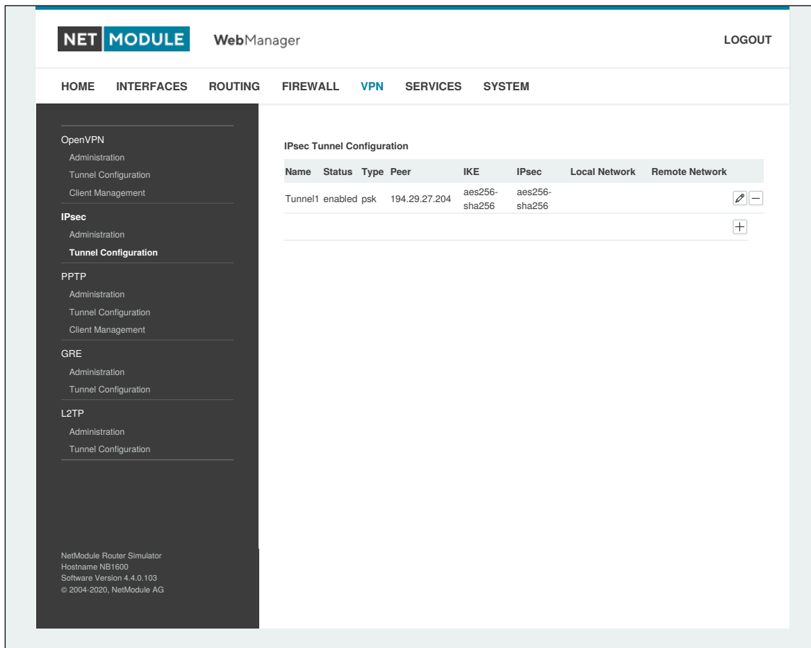
Abbildung 5.31.: IPsec-Konfiguration
