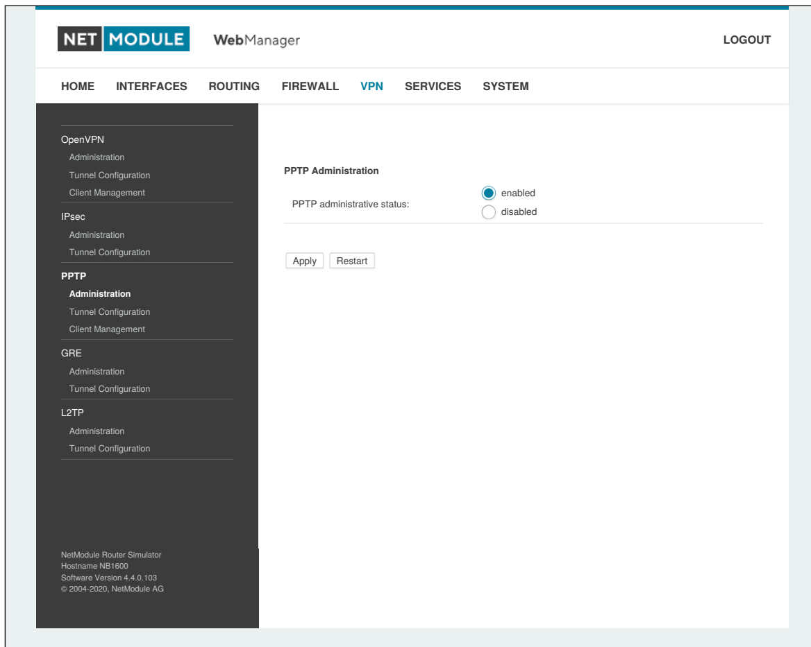
Abbildung 5.34.: PPTP-Verwaltung
