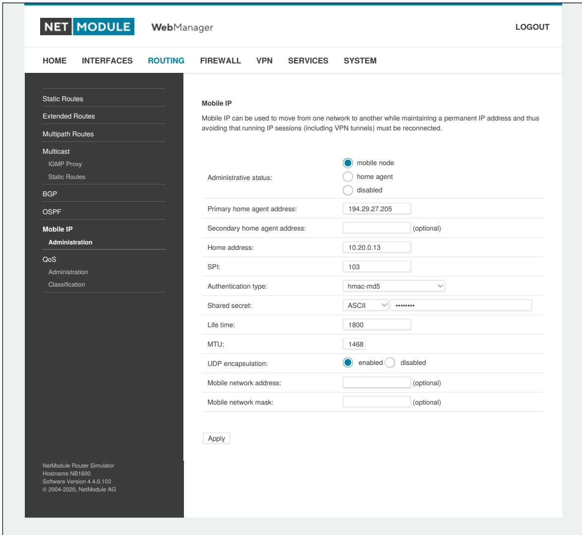
Abbildung 5.24.: Mobile IP
