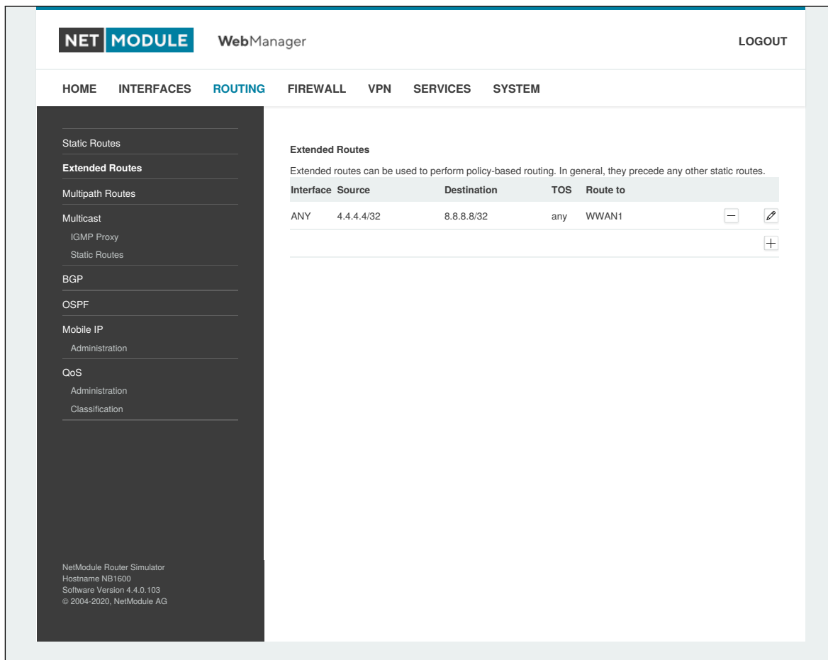
Abbildung 5.22.: Erweitertes Routing
