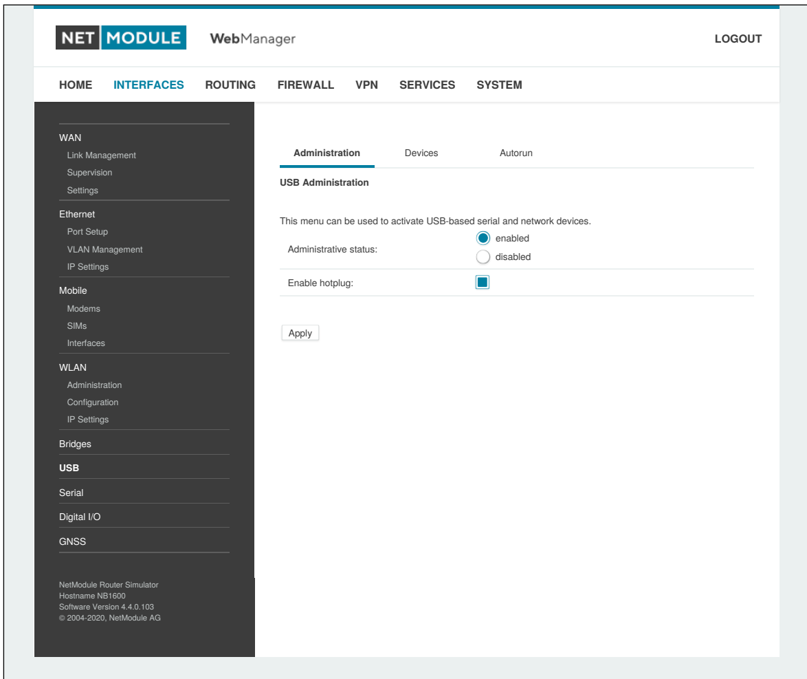
Abbildung 5.17.: USB-Verwaltung
