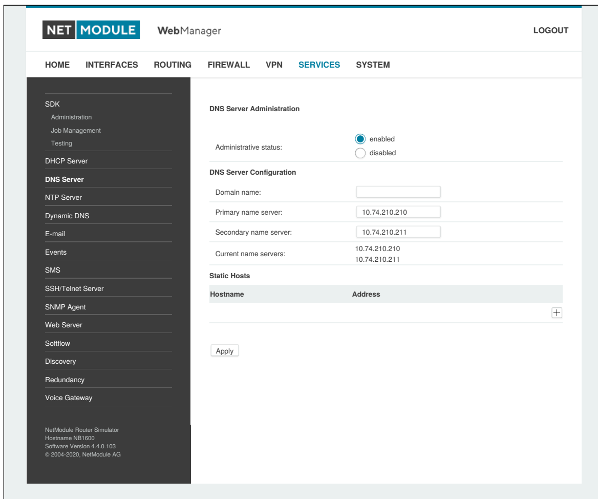
Abbildung 5.41.: DNS-Server
