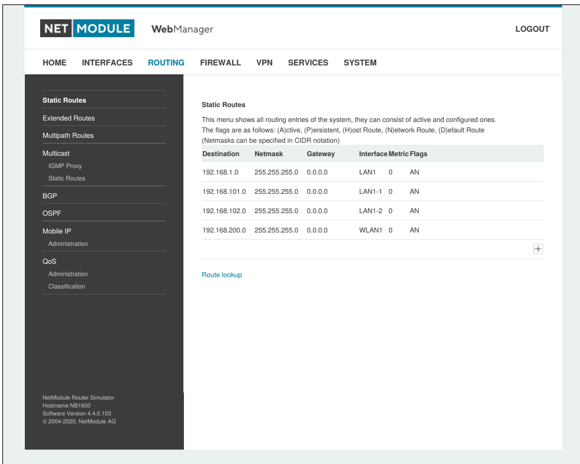
Abbildung 5.25.: Statisches Routing
