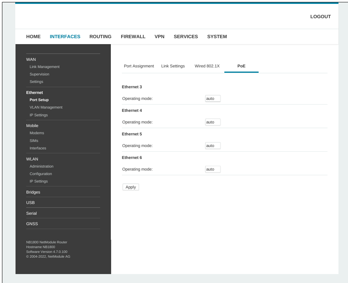
Abbildung 5.10.: PoE-Power-Supply
