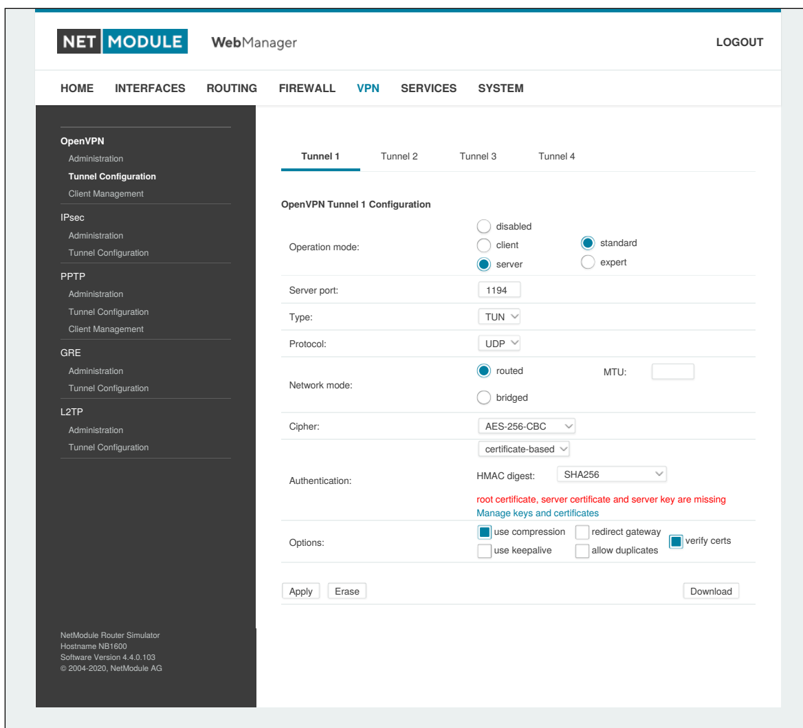
Abbildung 5.35.: Konfiguration von OpenVPN
