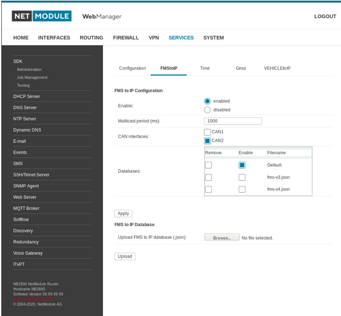
Abbildung 5.56.: ITxPT FMS-to-IP
