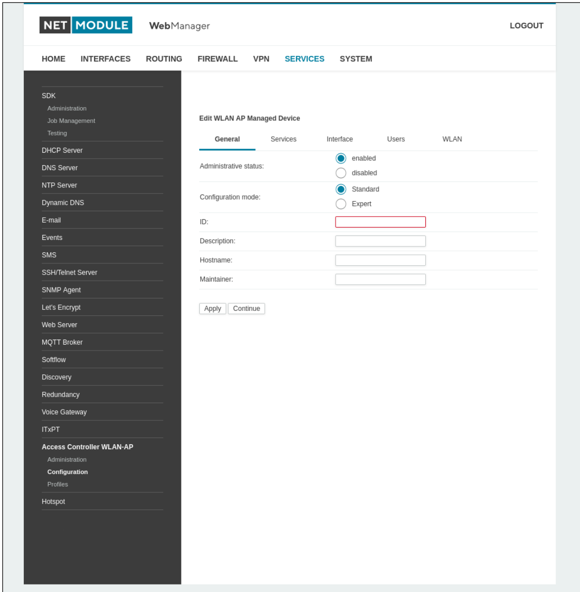
Abbildung 5.61.: AC WLAN-AP Configuration
