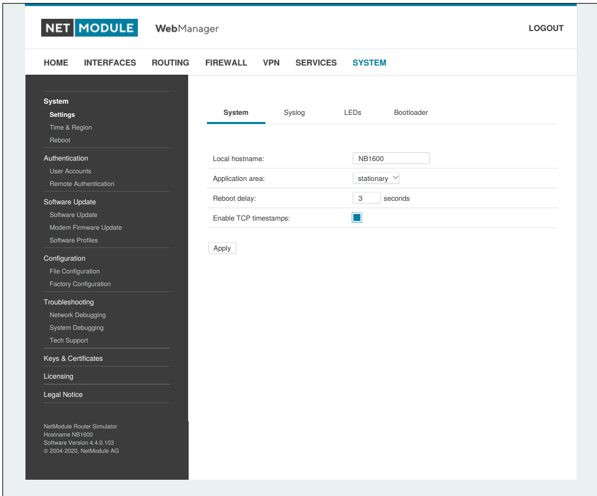
Abbildung 5.61.: System
