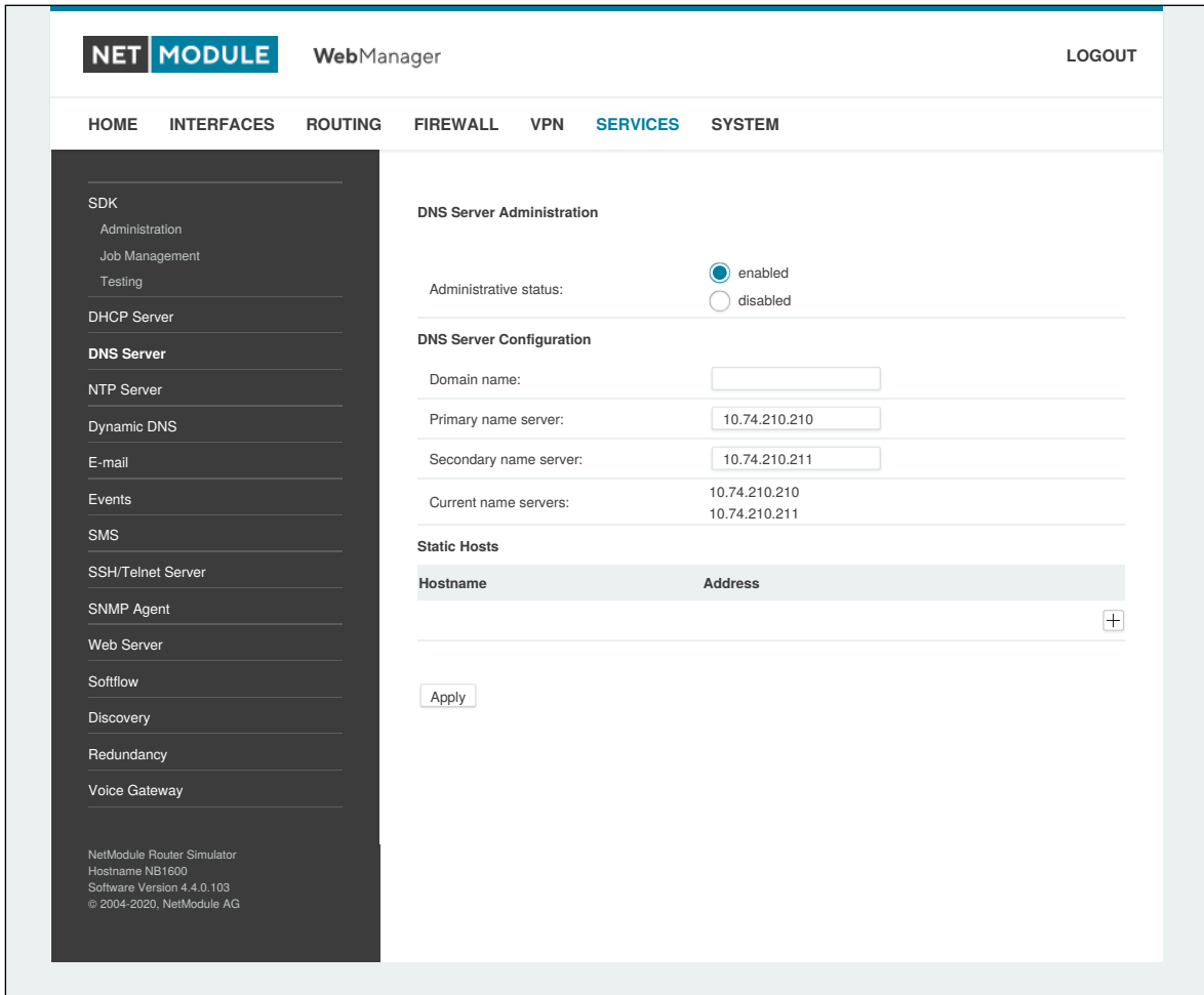
Abbildung 5.44.: DNS-Server
