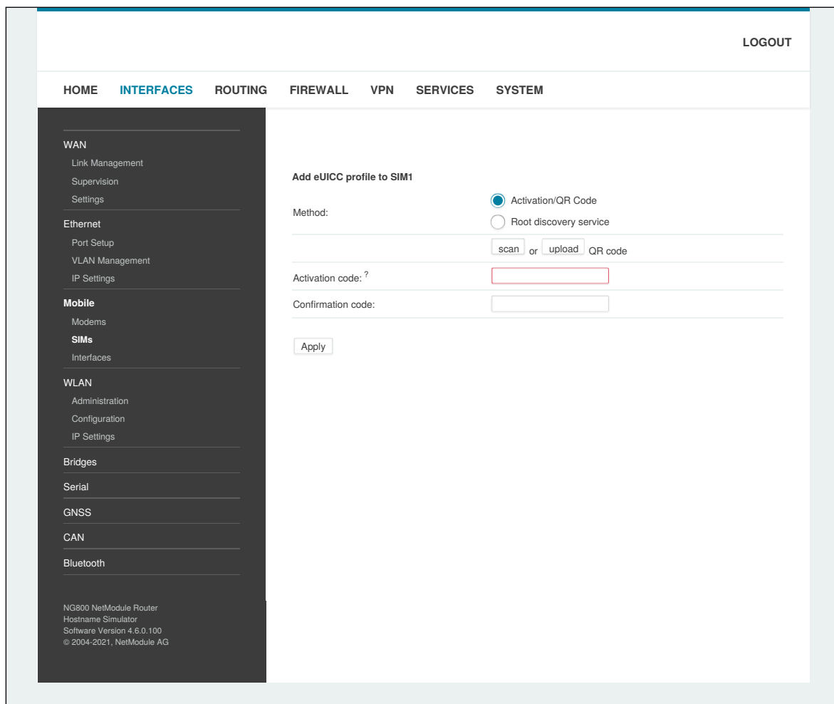
Abbildung 5.15.: eUICC-Profil hinzufügen
