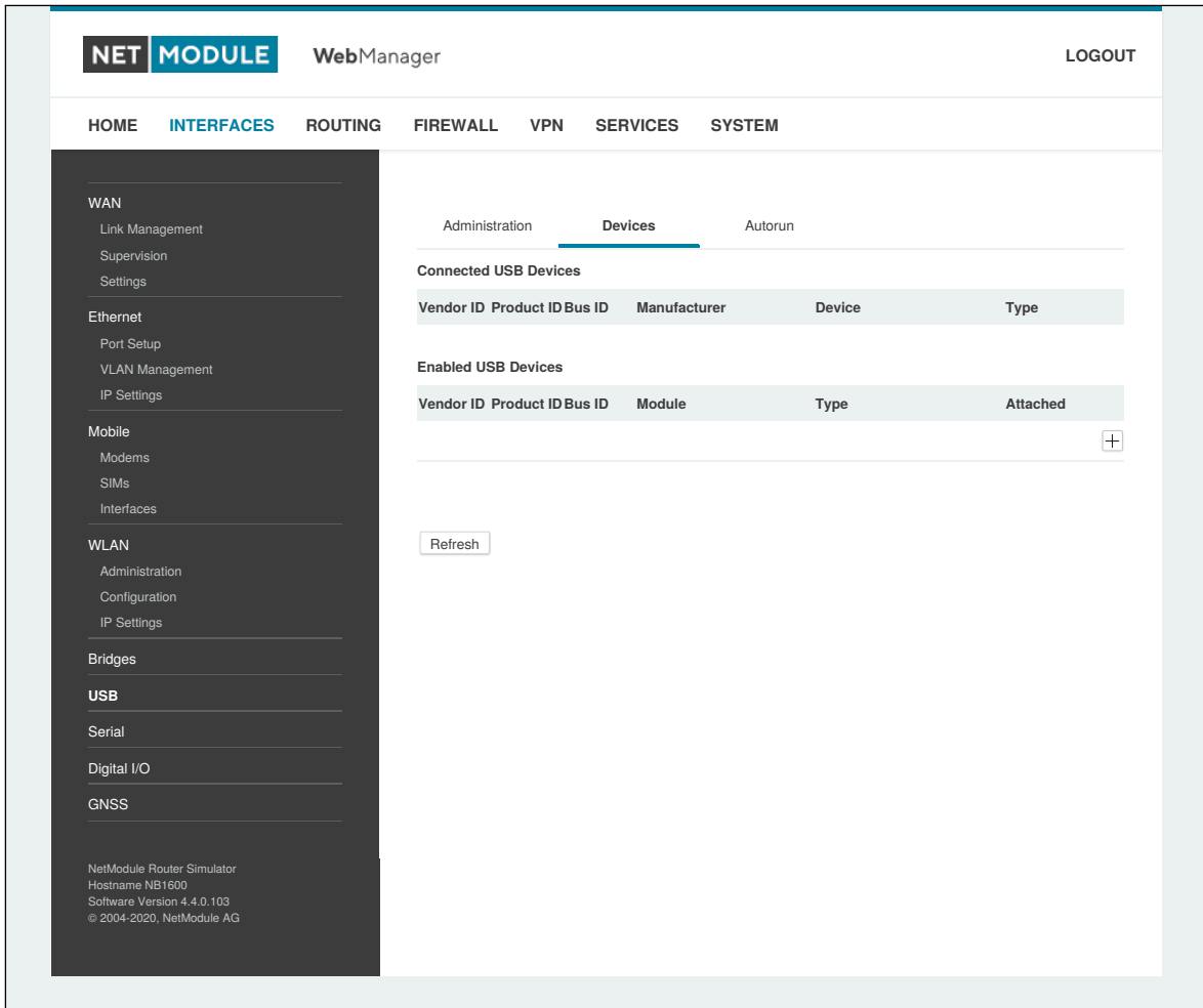
Abbildung 5.21.: USB-Geräteverwaltung
