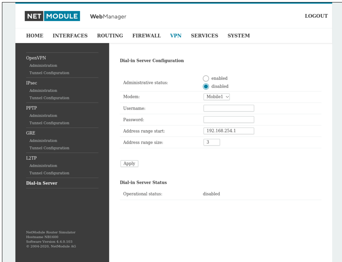
Abbildung 5.38.: Einwahlserver-Einstellungen
